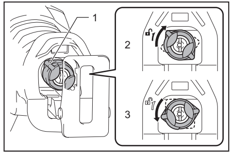
▶ 1. 날 클램프 레버 2. 풀린 위치 3. 고정 위치
