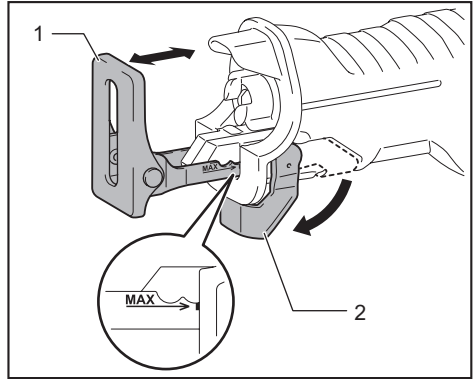
▶ 1. 슈 2. 슈 조절 레버
