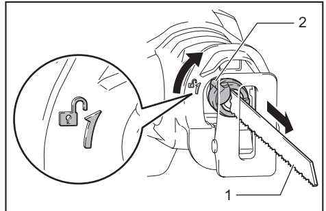
▶ 1. 컷소 날 2. 날 클램프 레버
