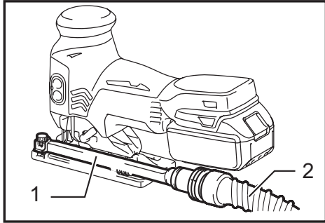
▶ 1. 더스트 노즐 2. 진공 청소기의 호스 그리고 더스트 노즐에 마귀다 진공 청소기를 연결합니다.
