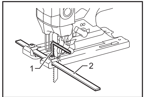
▶ 1. 볼트 2. 롤러 바
