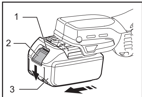
▶ 1. 적색 표시기 2. 버튼 3. 배터리 카트리지
