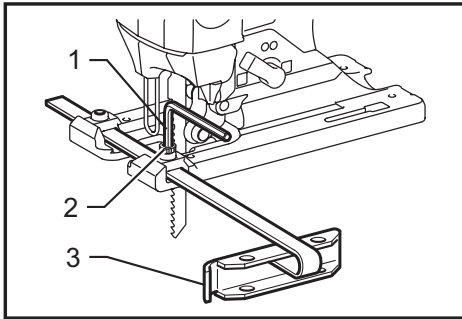
▶ 1. 육각 렌치 2. 볼트 3. 펜스 가이드
