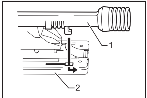
▶ 1. 더스트 노즐 2. 베이스
