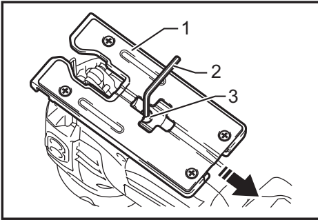
▶ 1. 베이스 2. 육각 렌치 3. 볼트
