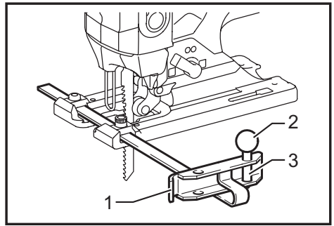
▶ 1. 펜스 가이드 2. 실 노브 3. 원형 가이드 핀
