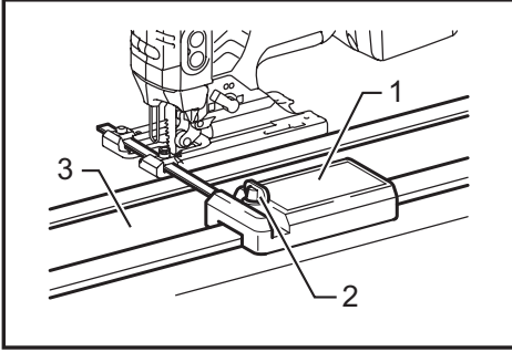
▶ 1. 가이드 레일 어댑터 2. 나사 3. 가이드 레일
