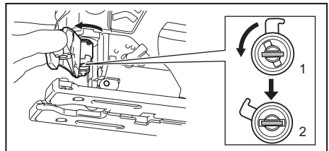
▶ 1. 고정 위치 2. 해제 위치
