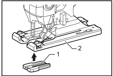
▶ 1. 분열 방지 장치 2. 베이스
