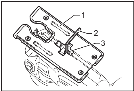
▶ 1. 베이스 2. 육각 렌치 3. 볼트 베이스를 기울이려면 육각 렌치로 베이스 뒤의 볼트를 풉니다. 베이스를 이동하면 베이스의 사선 구멍 중앙에 볼트가 위치하게 됩니다.
