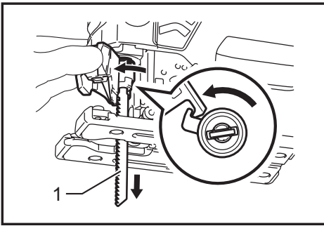
▶ 1. 직소 날
