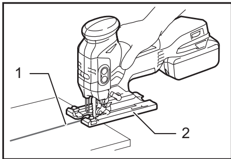
▶ 1. 절단선 2. 베이스 날이 다른 물체에 닿지 않은 상태에서 공구를 켜고 날이 전속력에 이를 때까지 기다립니다. 그리고 베이스를 작업물 위에 평평하게 놓고 미리 표시해 둔 선을 따라 공구를 움직입니다. 곡선을 자를 때는 공구를 천천히 움직입니다.
