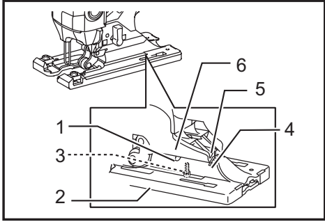
▶ 1. 사선 구멍 2. 베이스 3. 볼트 4. 등급 5. V 새김눈 6. 기어 틀
